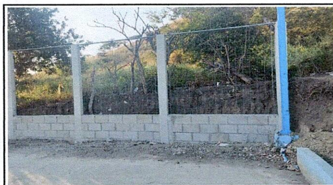
Foto 3: Mejoramiento de cercamiento perimetral: Colocación de 64 metros de electro malla
